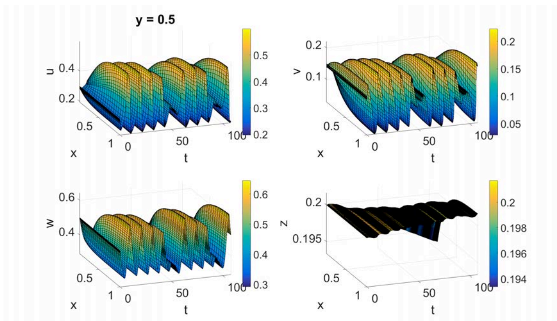
Рис.1. Залежність поверхневих покриттів СО u(x,y,t) , v(x,y,t) , частки поверхні неперевбудованої структури (1 \times 1) w(x,y,t) та ступеня огранювання z(x,y,t) при p_u = 2,65 \cdot 10^{-5} Торр, p_v = 6,4 \cdot 10^{-5} Торр та фіксованому значенні координати y = 0,5 .
