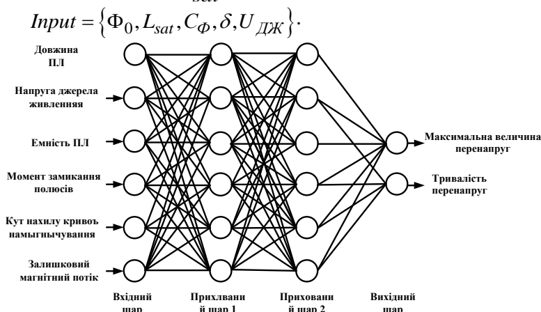
Рис. 1. Штучна нейронна мережа з архітектурою багатошарового перцептрону
