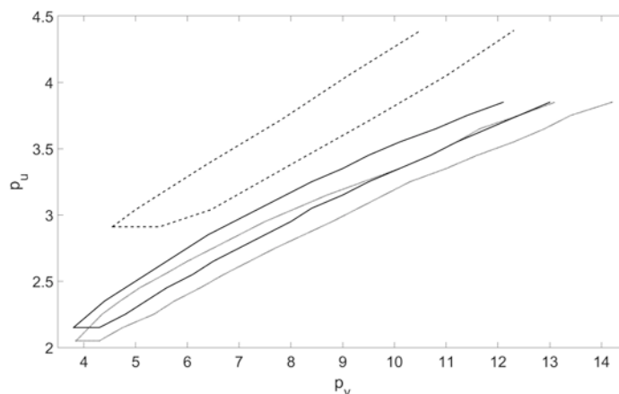
Рис.2. Діаграма стійкості реакції окислення СО в площині тисків (p_u, p_v) для двовимірної моделі (1)-(5) (суцільна лінія), двовимірної моделі без урахуванням огранювання [2] (пунктирна лінія) та одновимірної моделі [6] (штрихова лінія).
