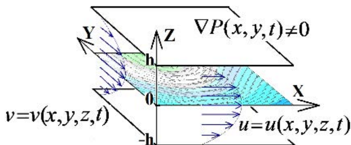
Рис.1. Схема течения
