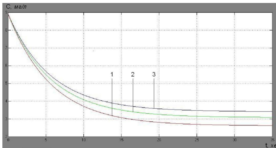
Рис.1. Зміна концентрації забруднення іонами нікелю на виході з коагулятора з часом при силі струму I = 0,5625 \text{ A} - крива 3, I_1 = 0,75 \text{ A} - крива 2, I_2 = 1 \text{ A} - крива 1
