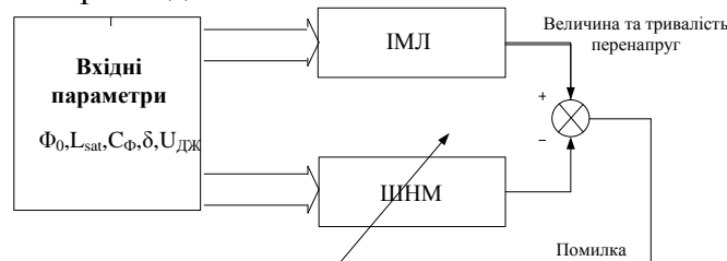
Рис. 2. Керуване навчання ШНМ
