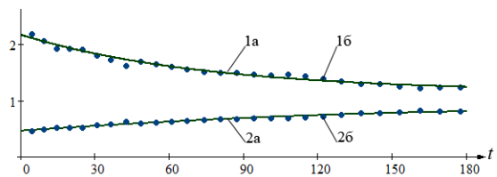
Рисунок 2. Результати експерименту 1: значення ЗЧ v_k – точковий графік 1а; оцінка ЗЧ v(t) – графік 1б; значення ЗП T_k – точковий графік 2а; оцінка ЗП T(t) – графік 2б.
